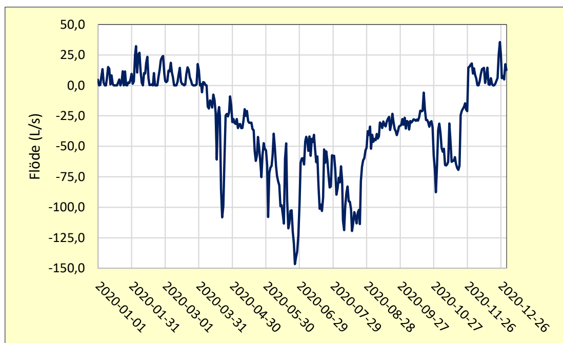
Figur 3. Totalt uttag och infiltration i akviferlagret under 2020. Sommardriftfallet, dvs med uttag från den ”kalla” sidan och infiltration på den ”varma” sidan representeras med negativa värden.
