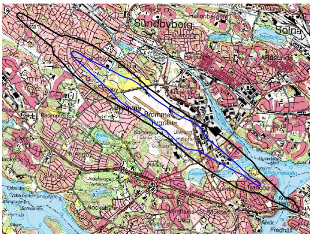
Figur 1: Bullerkurvan för maximal ljudnivå 80 dB(A) (svart), bullerkurvan för FBN 60 (blå) baserat på flygtrafiken 2017.
