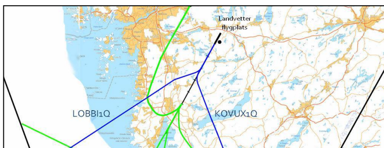
Figur 5. RNP-AR-procedurer LOBB1Q och KOVUX1Q för bana 03. Översta dragningar anger slutna P-RNAV STAR i befintligt system.
