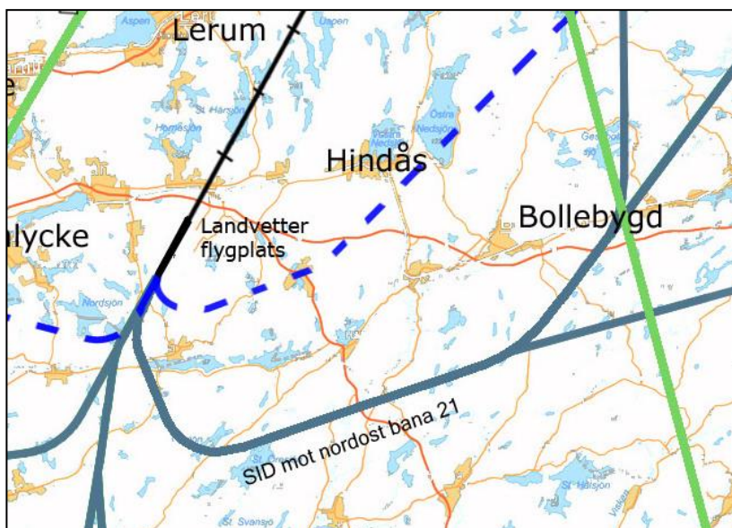
Figur 9. SID LABAN från bana 21 med särskild restriktion dag/kväll
