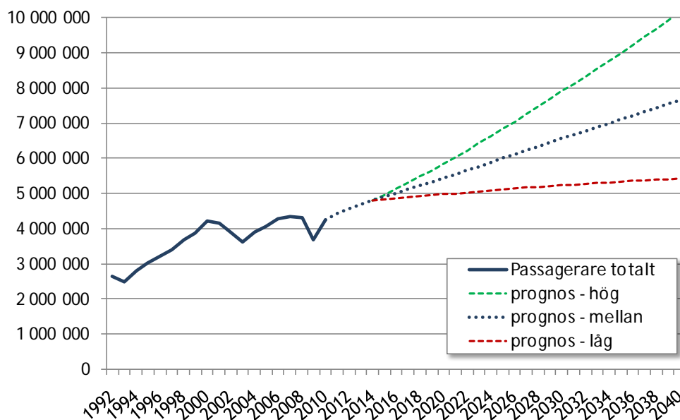
Figur 3 Passagerarprognos
